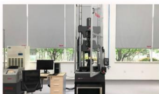
600kN液压万能试验机 用于金属材料的力学性能试验
